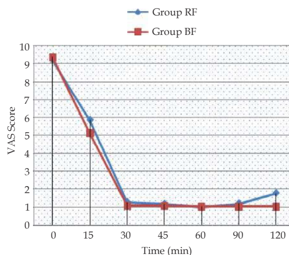
Fig. 1: VAS Scores.
